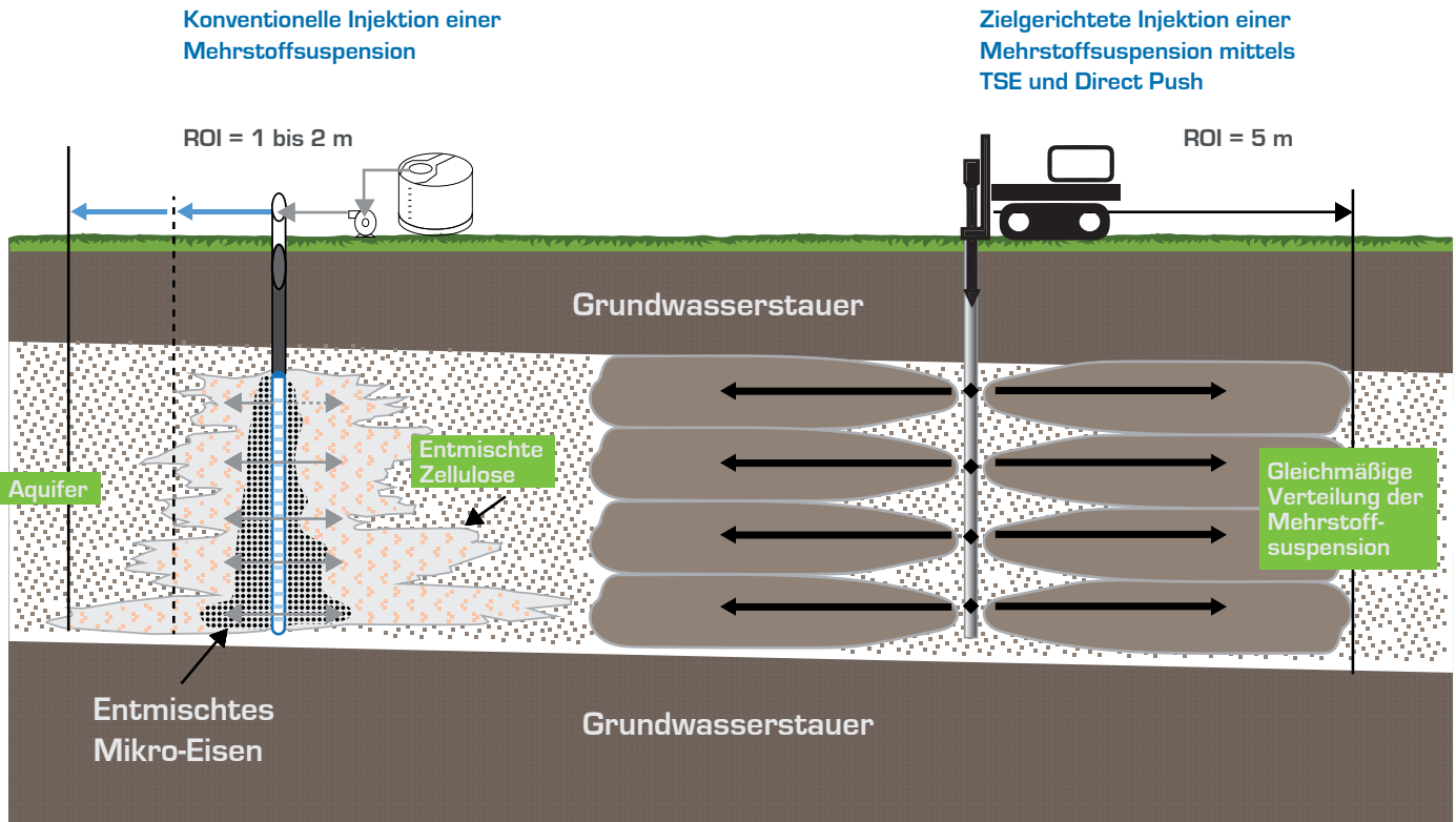
Vergleich von Injektion und Verteilung einer Mehrstoffsuspension (z.B. Mikro-Eisen und Zellulose) in einem Grundwasserleiter
